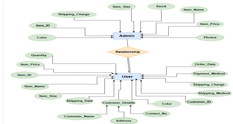
Figure 01- ER Diagram
